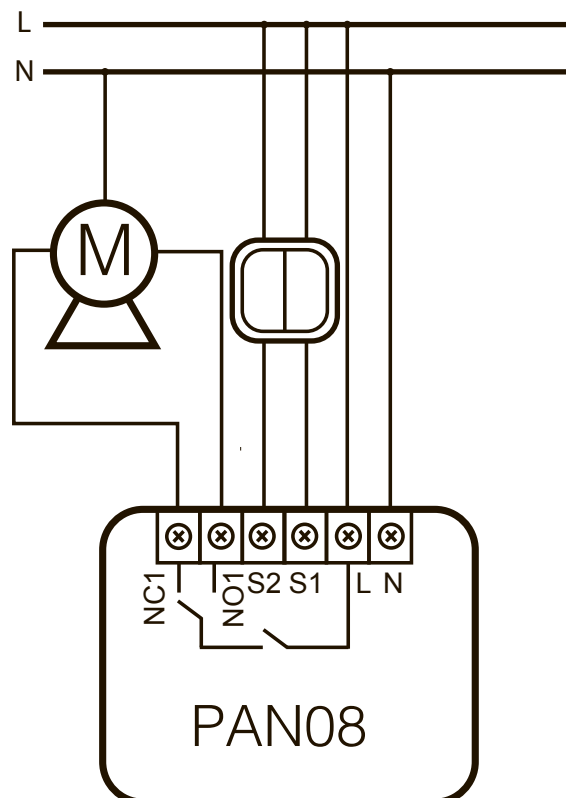
Рис. 1. Схема монтажа
